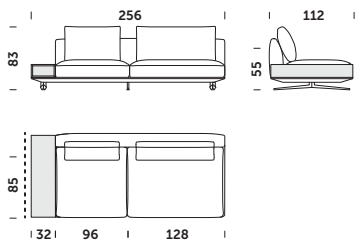
EOS_256 A 256x112x83cm
