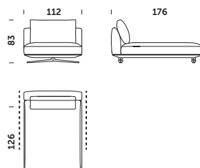
DB_176 B 112x176x83cm
