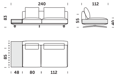
EOS_240 B 240x112x83cm
