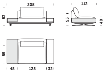
EO2S_208 A 208x112x83cm
