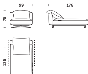
DB_176 C 99x176x83cm
