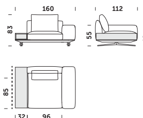
EKS_160 B 160x112x83cm
