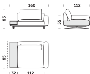
EKS_160 A 160x112x83cm
