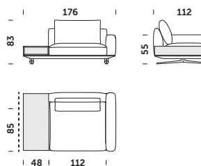
EKS_176 C 176x112x83cm
