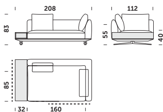
ENOS_208 A 208x112x83cm
