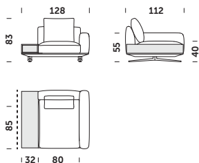
EKS_128 A 128x112x83cm
