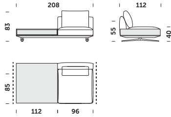
EODS_208 A 208x112x83cm
