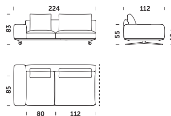
EK_224 A 224x112x83cm
