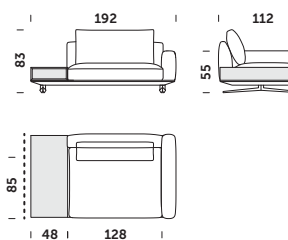
EKS_192 B 192x112x83cm
