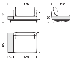
EKS_176 A 176x112x83cm
