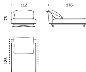
DB_176 D 112x176x83cm
