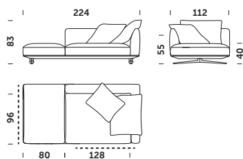
ENO_224 D 224x112x83cm
