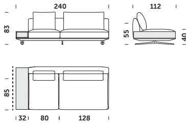
EOS_240 A 240x112x83cm
