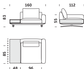
EKS_160 C 160x112x83cm
