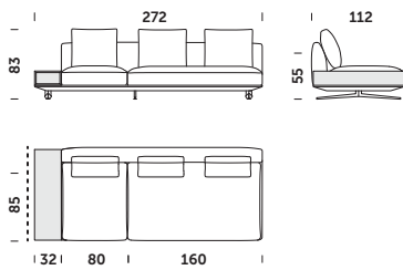
EOS_272 A 272x112x83cm
