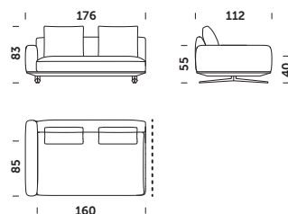
EK_176 A 176x112x83cm
