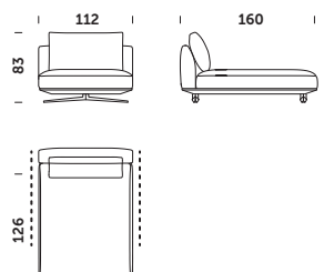
DB_160 B 112x160x83cm
