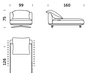
DB_160 C 99x160x76cm
