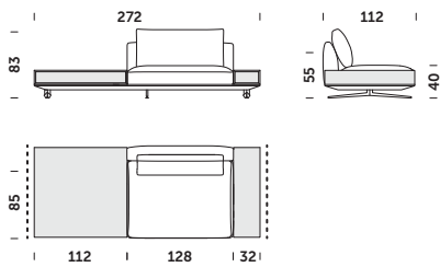
EODS_272 A 272x112x83cm
