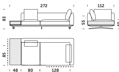
ENOS_272 C 272x112x83cm
