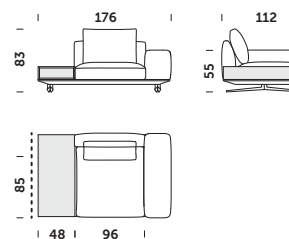
EKS_176 D 176x112x83cm
